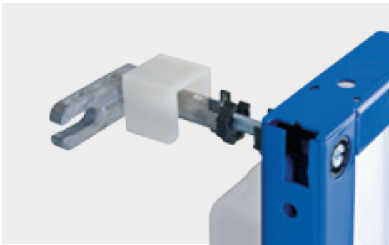
↑ Wandbevestiging om installatie-elementen aan de wand te verankeren. Comfortabele en nauwkeurige diepte verstelling vanaf de voorkant.
