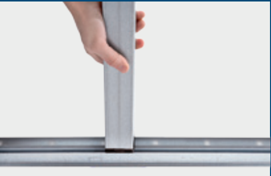
↑ Bevestig de ruimtehogestanders aan het plafond vast en schuif hem uit naar onderen. Klik de stander in het Geberit Duofix systeempromiel.
